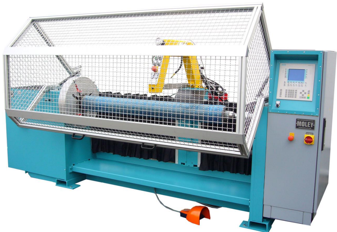
MOLEY®-Standard 500/1600
